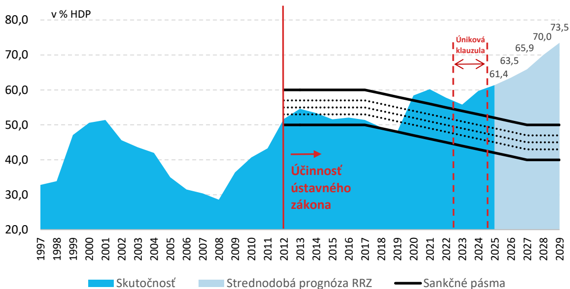
Graf 4: Vývoj hrubého dlhu verejnej správy
