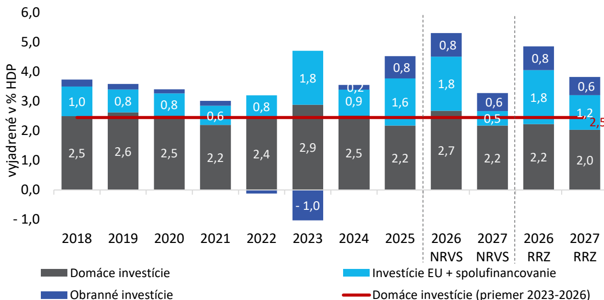
Graf 2: Štruktúra verejných investícií – dlhodobé trendy a výhľad pre rok 2027
