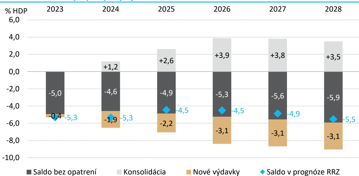
Graf 6: Kumulatívne príspevky k vývoju salda VS v aktuálnom volebnom období
