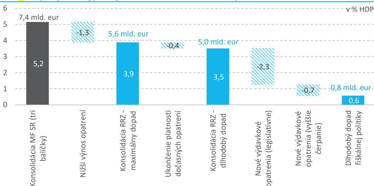
Graf 5: Príspevky fiškálnej politiky od roku 2023 na odhadované hospodárenie v roku 2028
