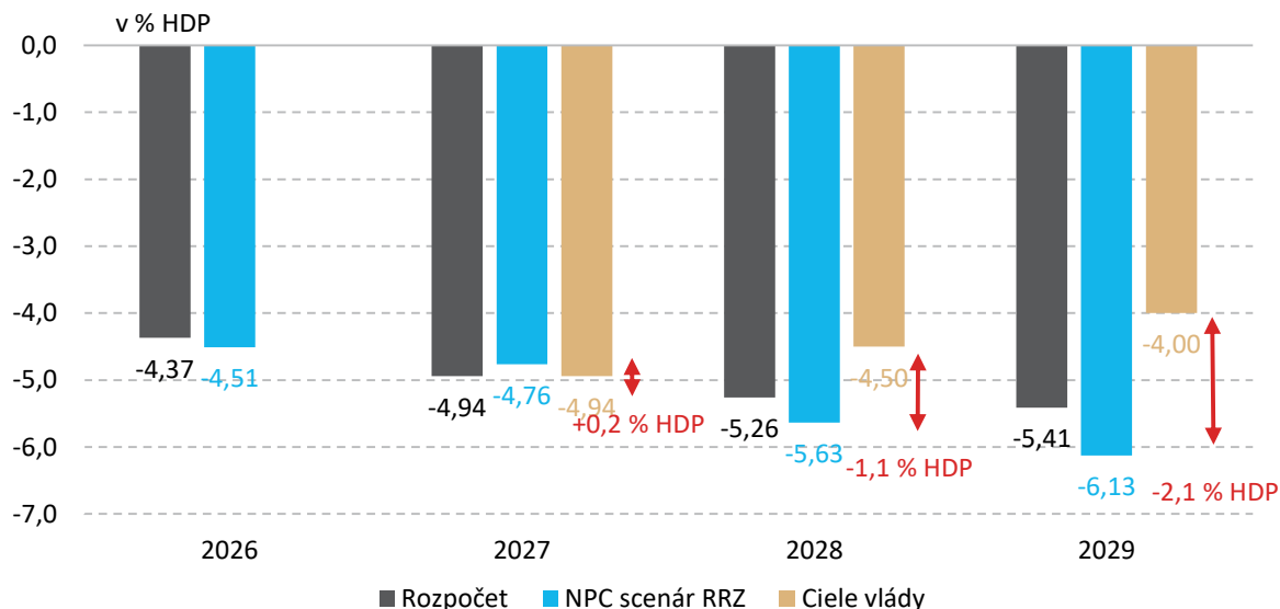
Graf 1: Rozpočtovaný vývoj salda VS oproti scenáru nezmenených politík podľa RRZ
