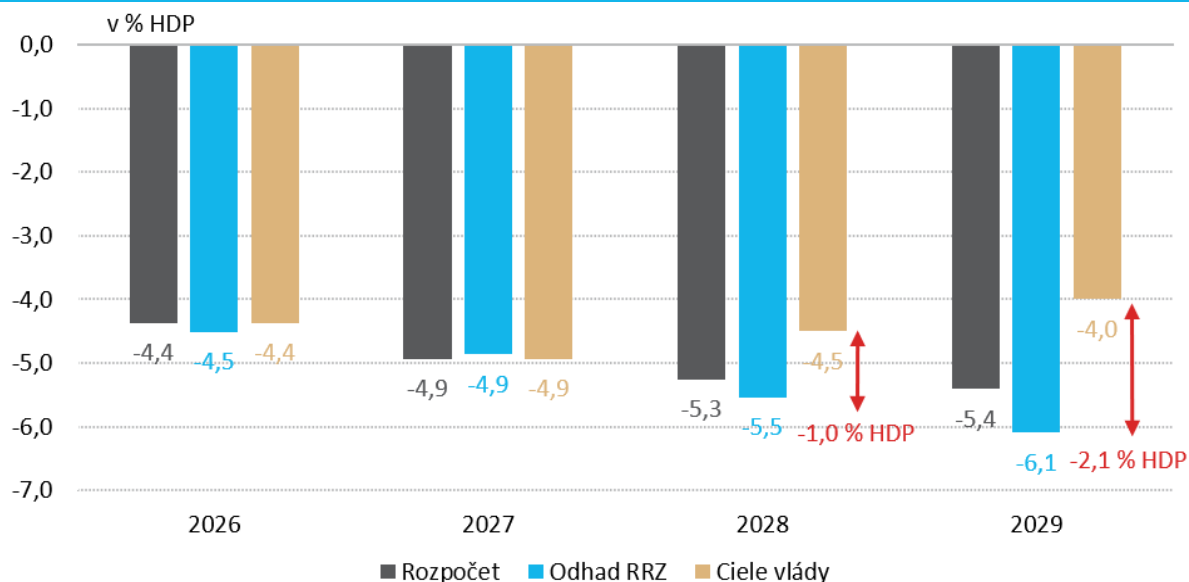
Graf 3: Odhad salda hospodárenia VS v rokoch 2026 až 2029 podľa RRZ a MF SR
